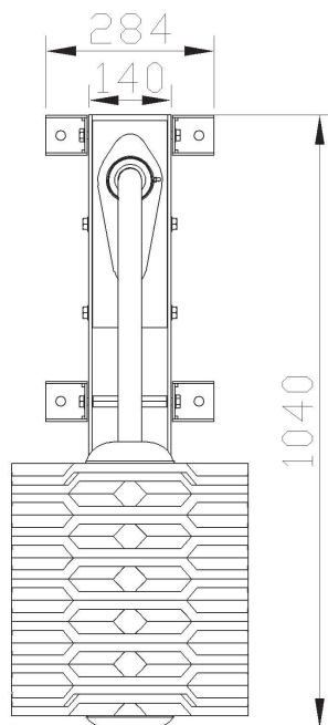
Midi 700381247 (284 x 1040 mm)
