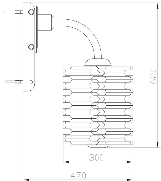
Mini 700381248 (470 x 620 mm)
